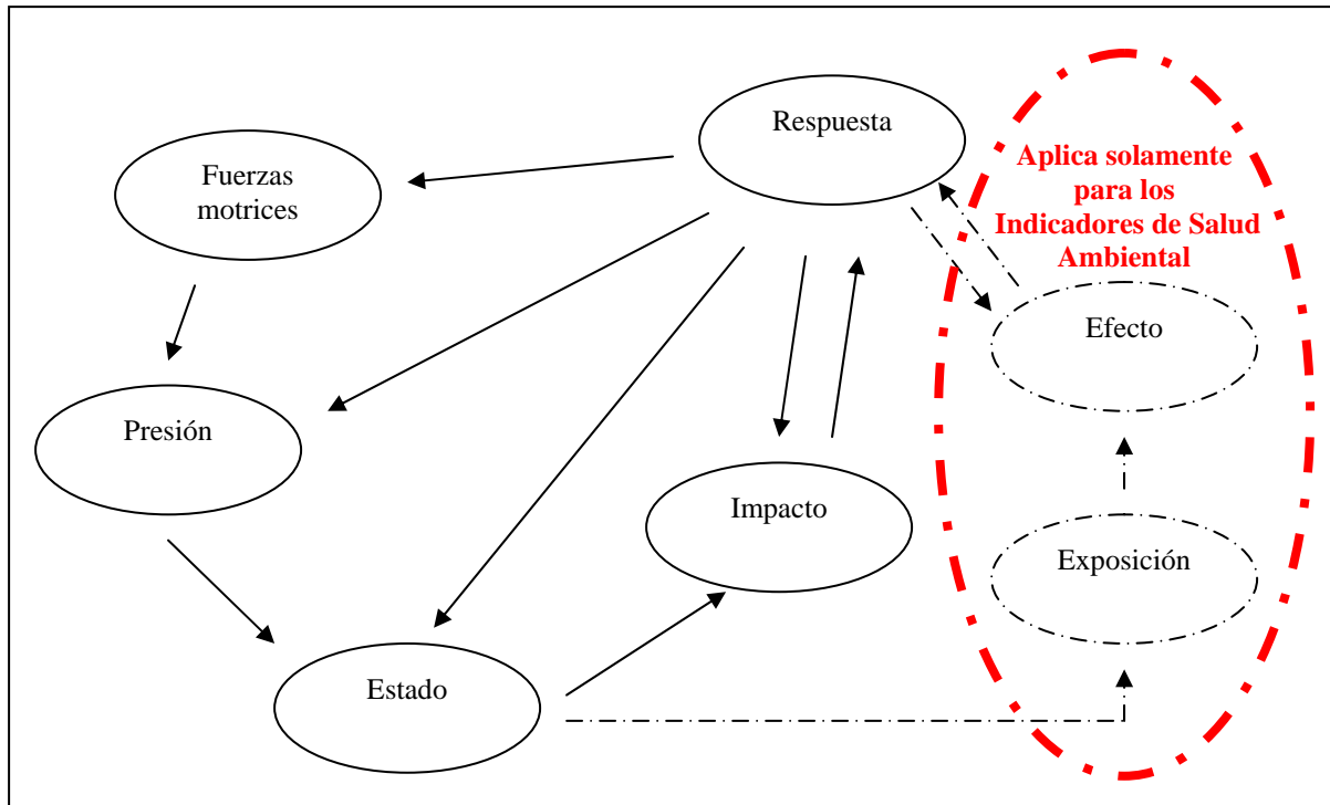
Figura 1: Modelo DPSIR
